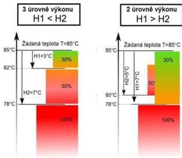
Obrázek 4. Hystereze H1 a H2 modulační výkonu
