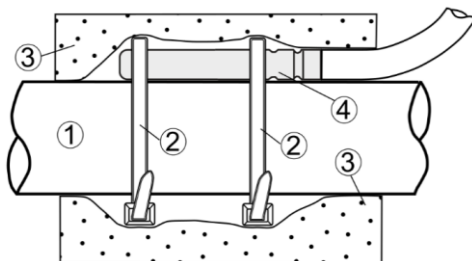
Obrázek 11. Instalace teplotního čidla na trubku, kde je: 1 - trubka, 2 - spona, 3 - tepelná izolace, 4 – teplotní čidlo
