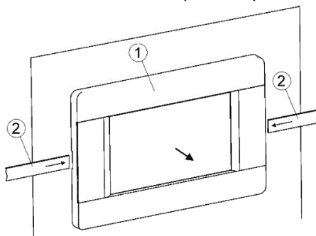
Obrázek 15. Demontáž ovládacího panelu
