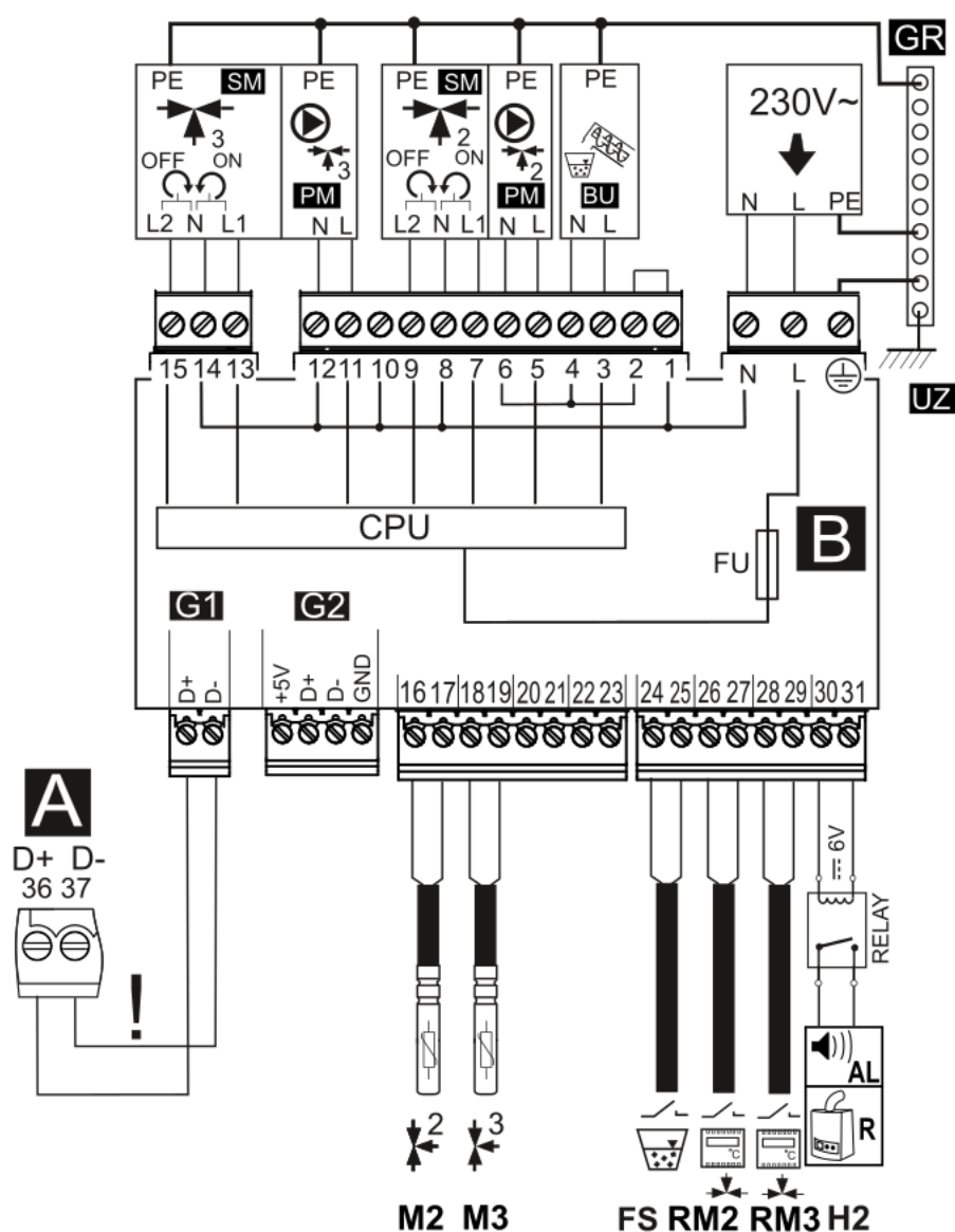
Obrázek 9. Elektrické schéma zapojení modulu B
