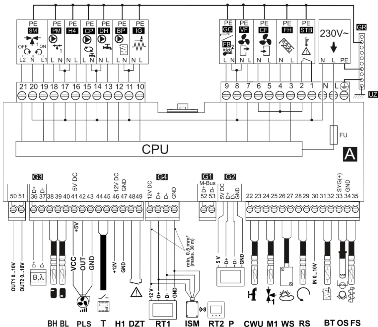
Obrázek 8. Elektrické schéma zapojení modulu A
