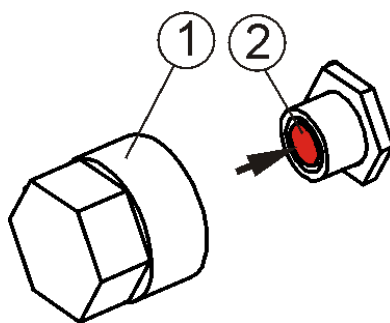
Obrázek 14. Resetování havarijního termostatu,
