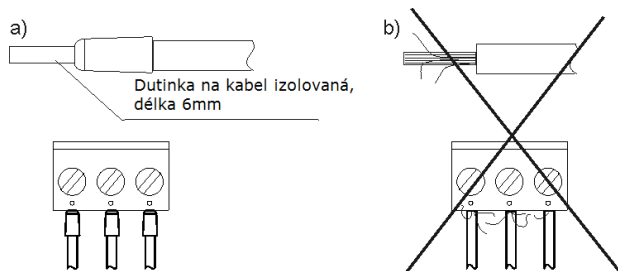
Obrázek 10. Připojení vodičů na svorky kde: a) správné připojení; b) špatné připojení
