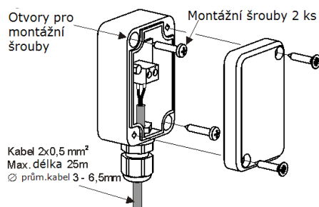
Obrázek 12. Připojení venkovního čidla CT6-P
