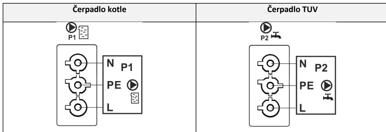
Obrázek 24. Elektrické schéma zapojení čerpadla kotle a čerpadla TUV
