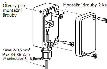
Obrázek 22. Připojení čidla venkovní teploty CT10P (není v základní výbavě kotle)
