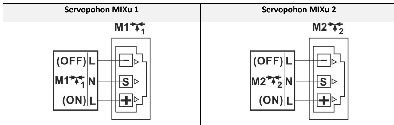
Obrázek 26. Elektrické schéma zapojení servopohonů MIXu
