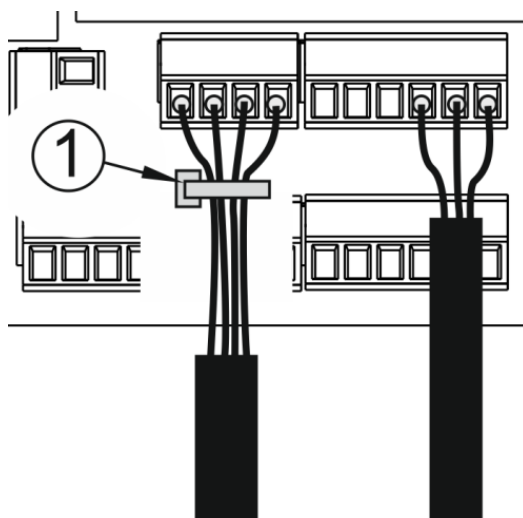
Obrázek 13. Délka odizolování kabelů, kde: 1 – kabelová páska
