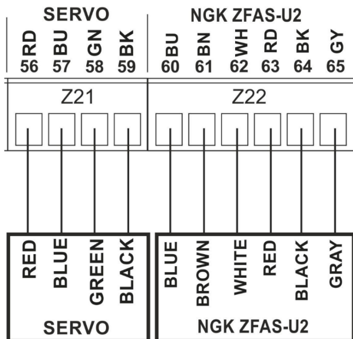
Obrázek 17. Elektrické schéma zapojení lambda sondy (NGK ZFAS-U2) a krokového motoru (SERVO)
