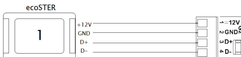
Obrázek 27. Čtyřvodičové připojení pokojového panelu ecoSTER
