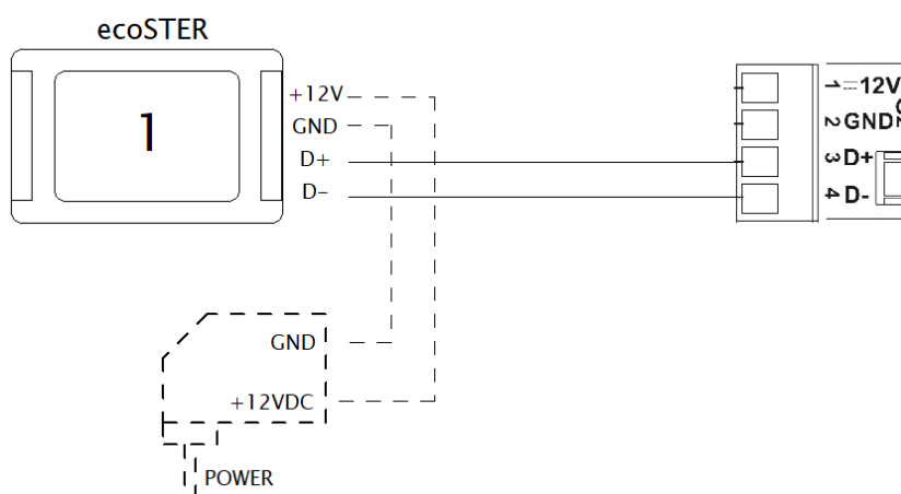
Obrázek 28. Dvouvodičové připojení pokojového panelu ecoSTER
