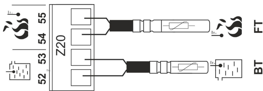
Obrázek 21. Připojení teplotních čidel,
