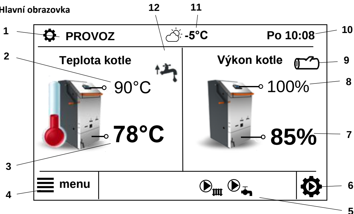
Obrázek 1. Hlavní obrazovka regulátoru
