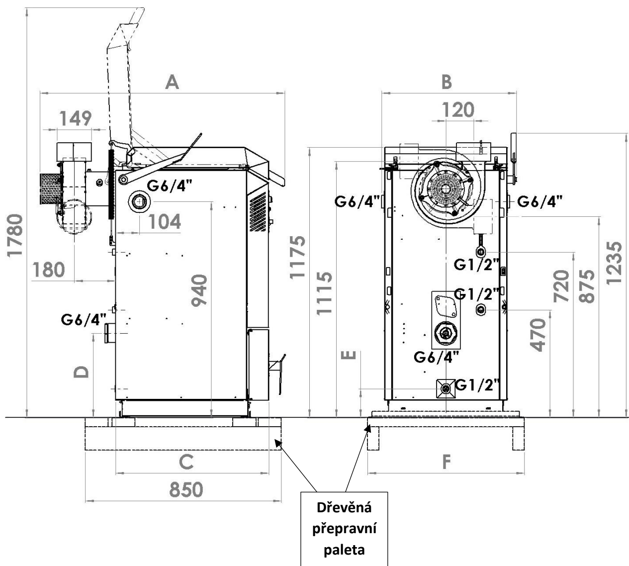
Tabulka základních rozměrů kotle BLAZE GREEN
